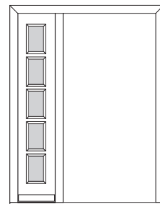
STM-Glimmer in Ausführungs-Variante 1 (AV1)
